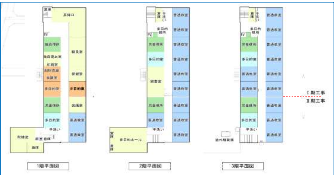
<増築校舎（Ⅱ期）平面図1～3階>
