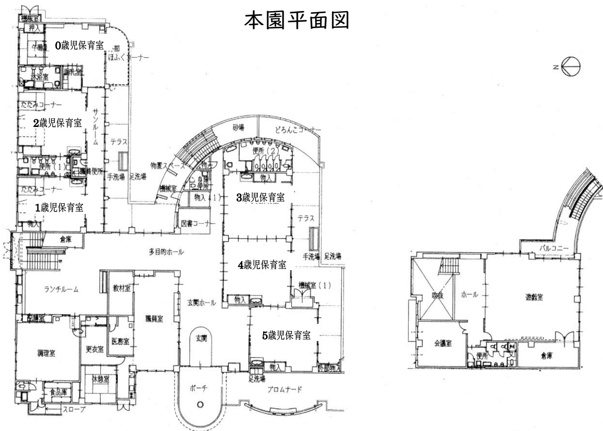
1階平面図
