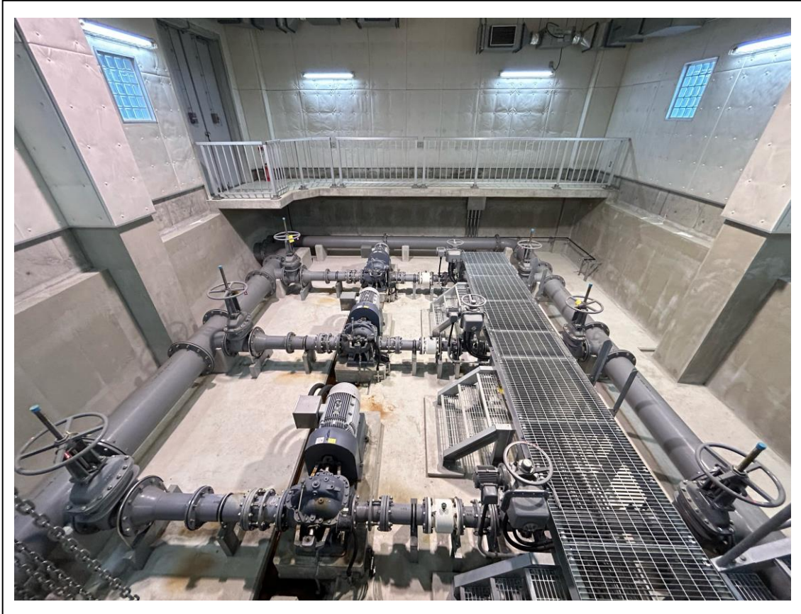
配水池の加圧ポンプ設備
