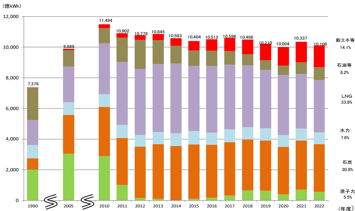
グラフ7：発受電電力量の推移
