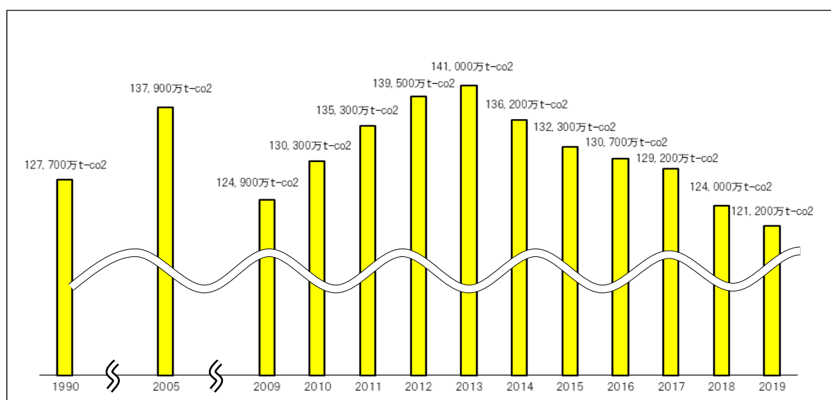
グラフ8：我が国の温室効果ガス排出量
