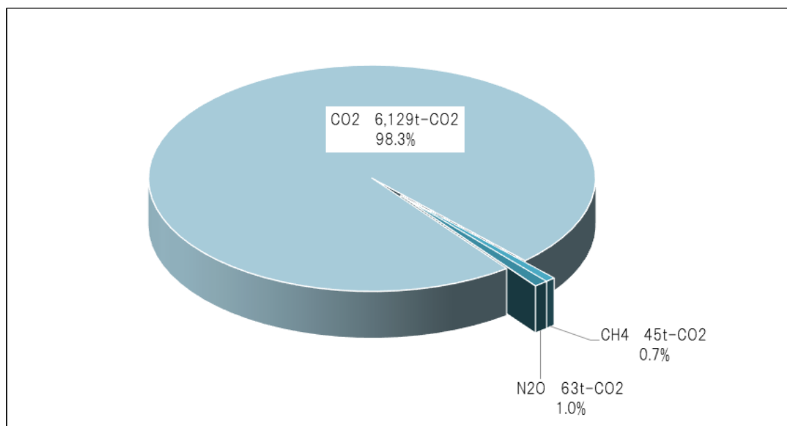
グラフ 4：2020 年度の温室効果ガスの種類別の排出状況
