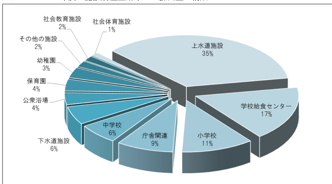
グラフ6：2020年度の施設別温室効果ガス排出量の構成
