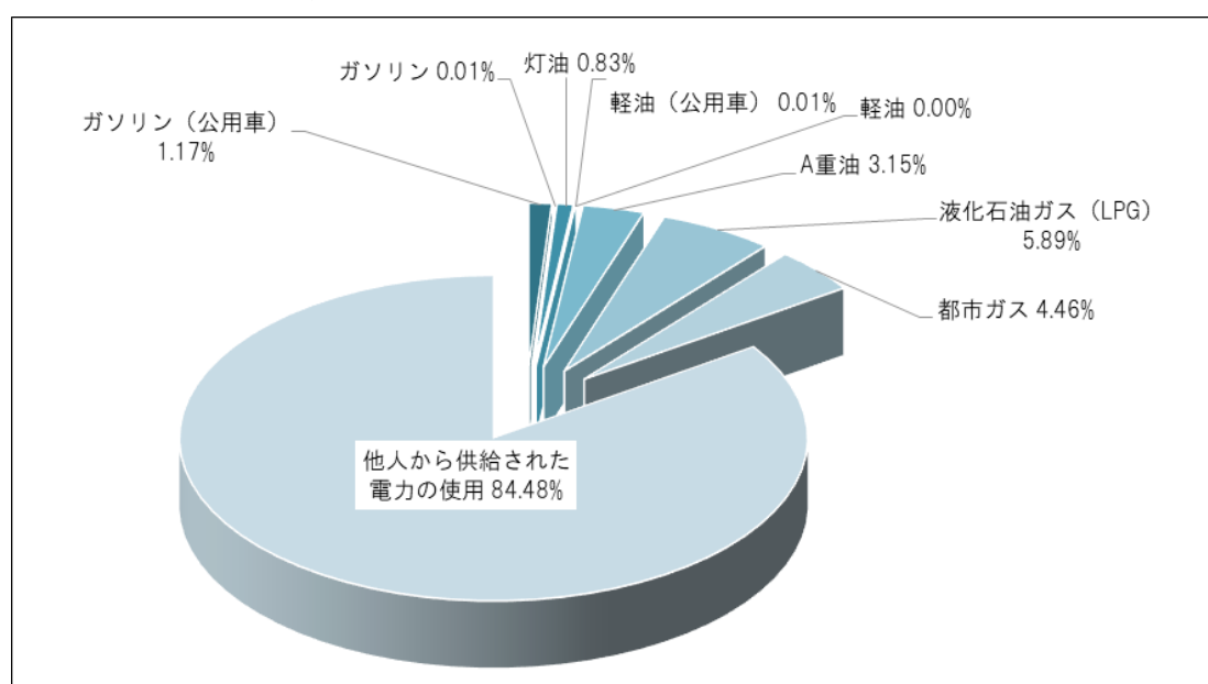
グラフ5：2020年度の燃料・電力の使用による二酸化炭素の排出状況
