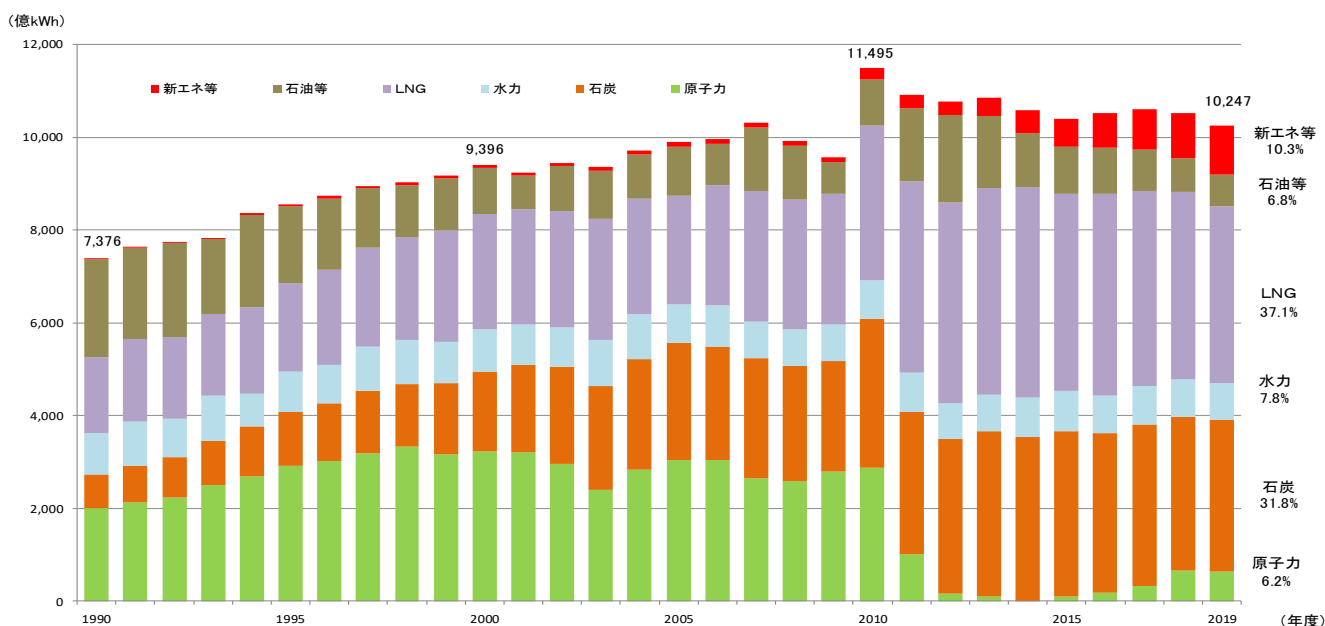
グラフ7：発受電電力量の推移
