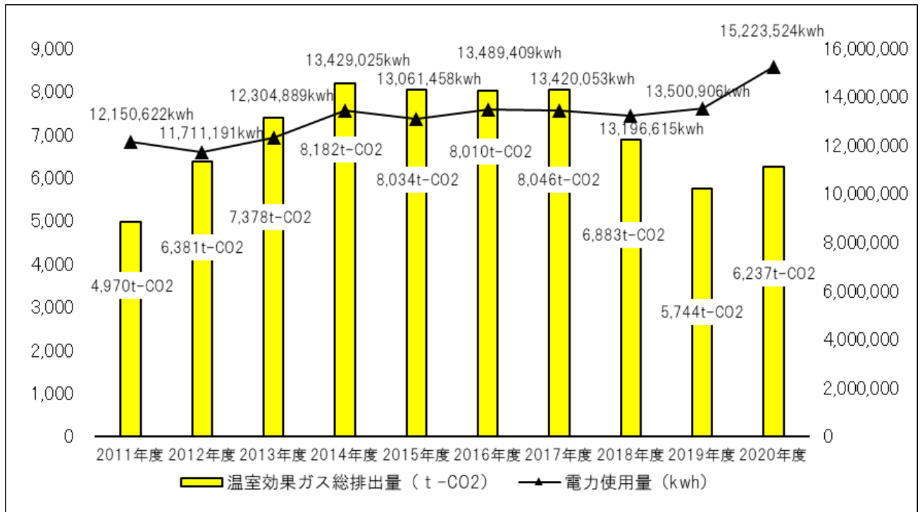
グラフ3：電力使用量と温室効果ガス総排出量の推移
