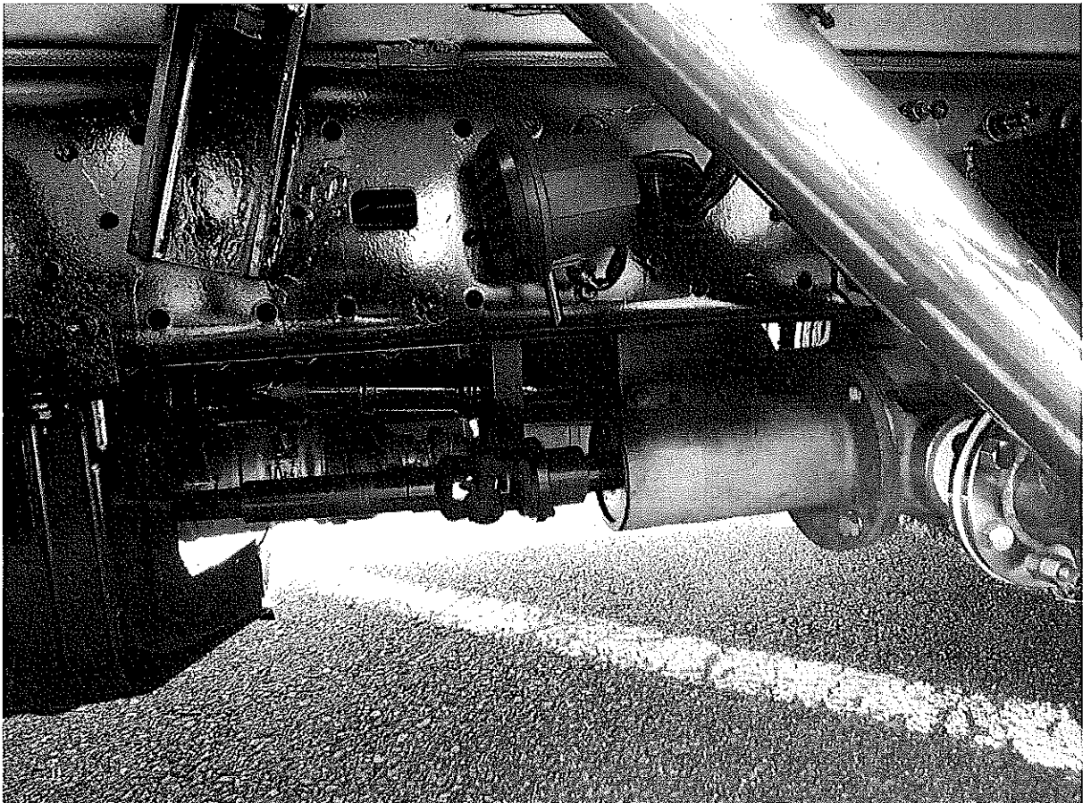
給水車の加圧ポンプにエンジンの動力を供給
