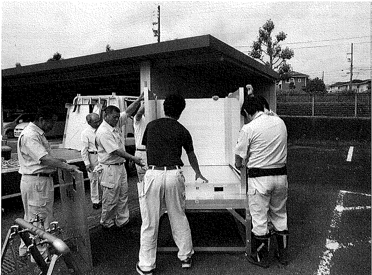
仮設給水タンクの組立②
