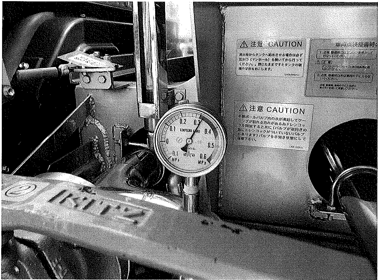
給水車の加圧ポンプで約0.3Mpaまで加圧
