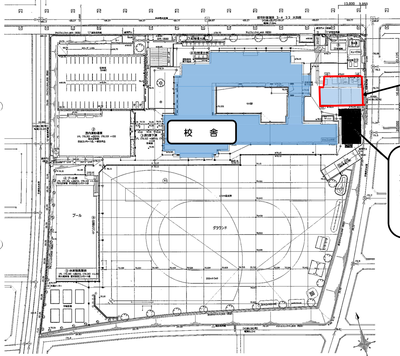
全体配置図 S=1:1000
