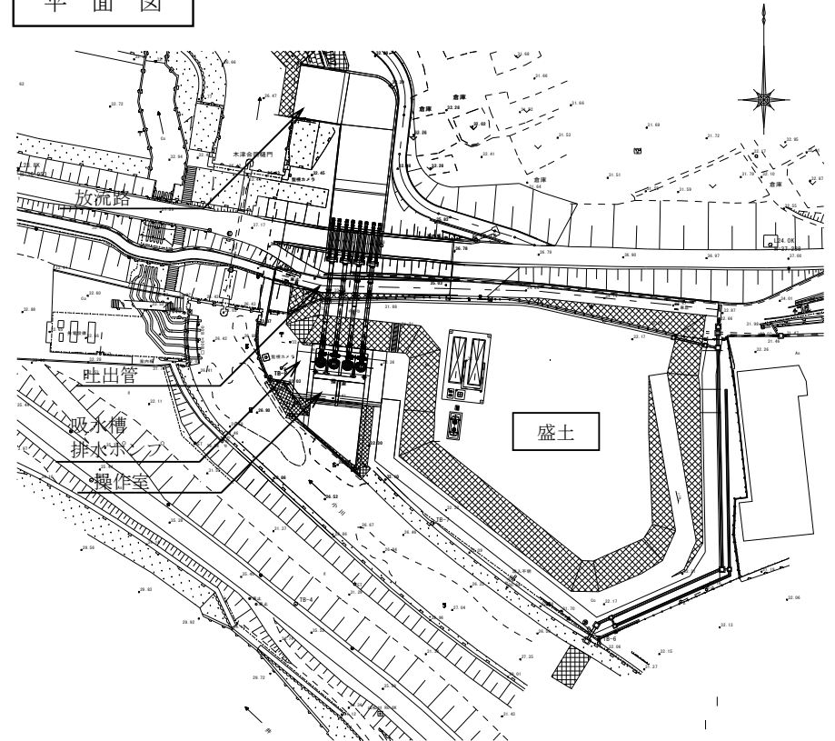
平面図
