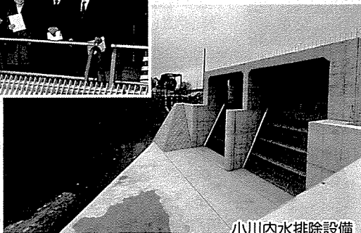
小川内水排除設備
