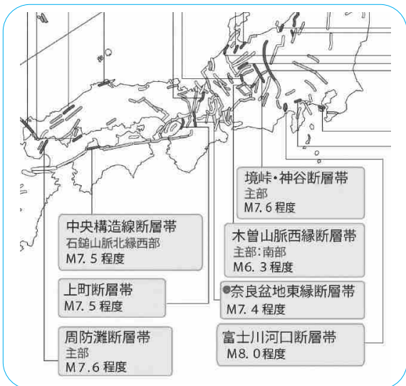
主要活断層の調査結果 (地震調査研究推進本部・7年1月15日公表)
